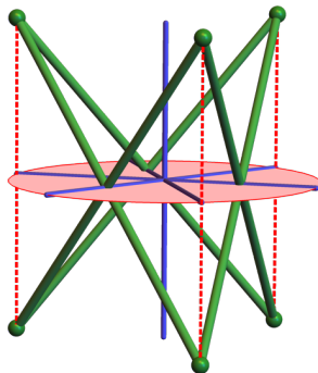
star D_{3h} (12)
